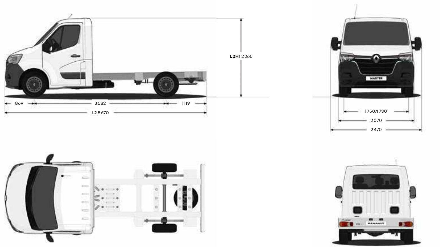
Pesos y cargas del chasis tracción simple cabina (kg)
